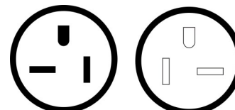
NEMA 6-20R NEMA 6-20P
